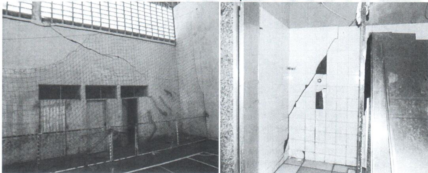
Rachaduras interior da quadra e vestiário
